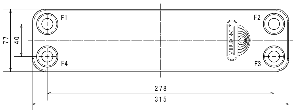
■ 寸法表
